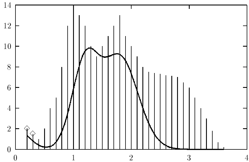
Figure 13.6: Où les paramètres des gaussiennes ne représentent plus la projection. Les losanges indiquent les valeurs modifiées par rapport à la fonction de la figure 13.5.
