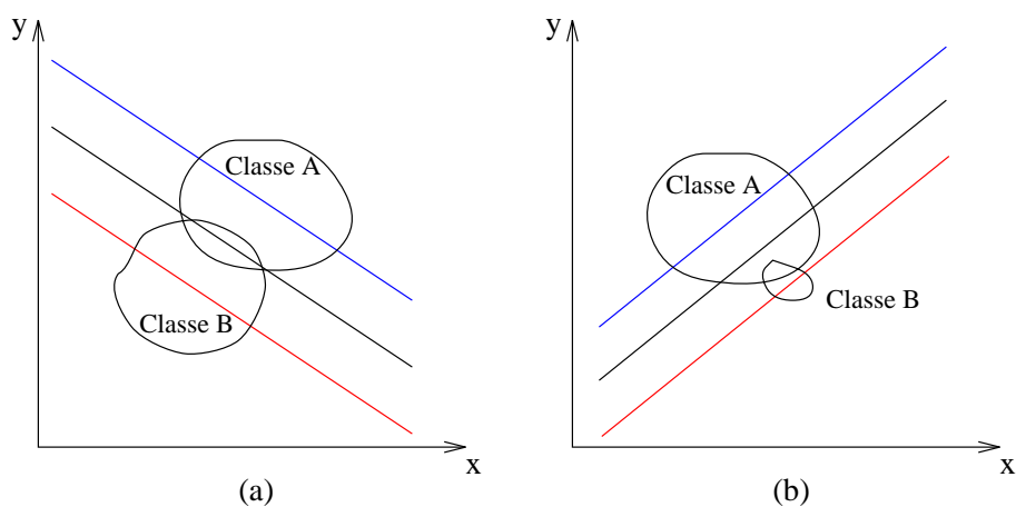
Figure 5.10: Solutions obtenues avec l'Adaline dans les situations illustrées par la figure 5.3. La ligne bleue (respectivement rouge) désigne la droite des moindres carrés de la classe A (respectivement B). Contrairement au Perceptron , l'Adaline détermine une solution lorsque le problème n'est pas linéairement séparable. Cette dernière minimisant le critère d'erreur quadratique, nous la considérons optimale.
