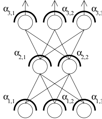
Figure 10.1: Perceptron multicouche avec les coefficients \alpha_{l,j}
