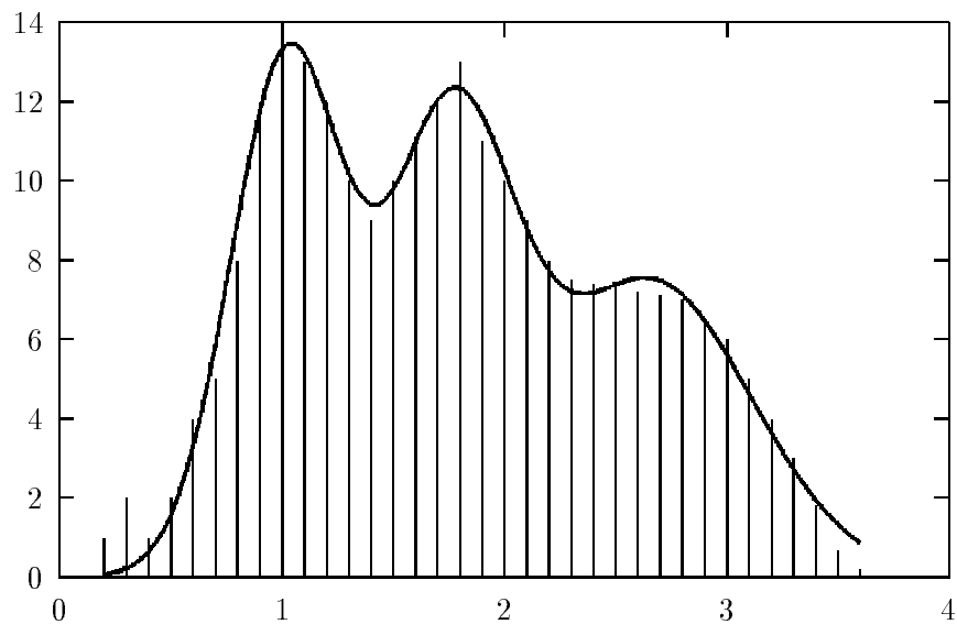
Figure 13.5: Une projection et son approximation par une somme de trois noyaux gaussiens
