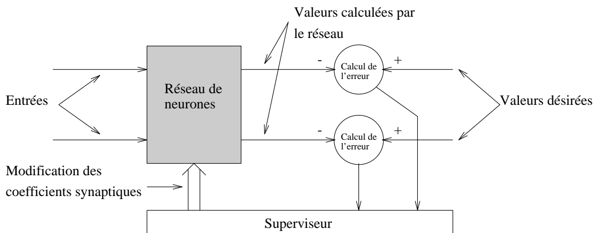
Figure 4.3: Apprentissage supervisé
